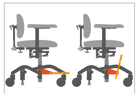
Oppfellbar fotplate gir god støtte ved høyere sitteposisjoner. Fotplaten felles innunder seteputens framkant og er da helt ute av veien.
